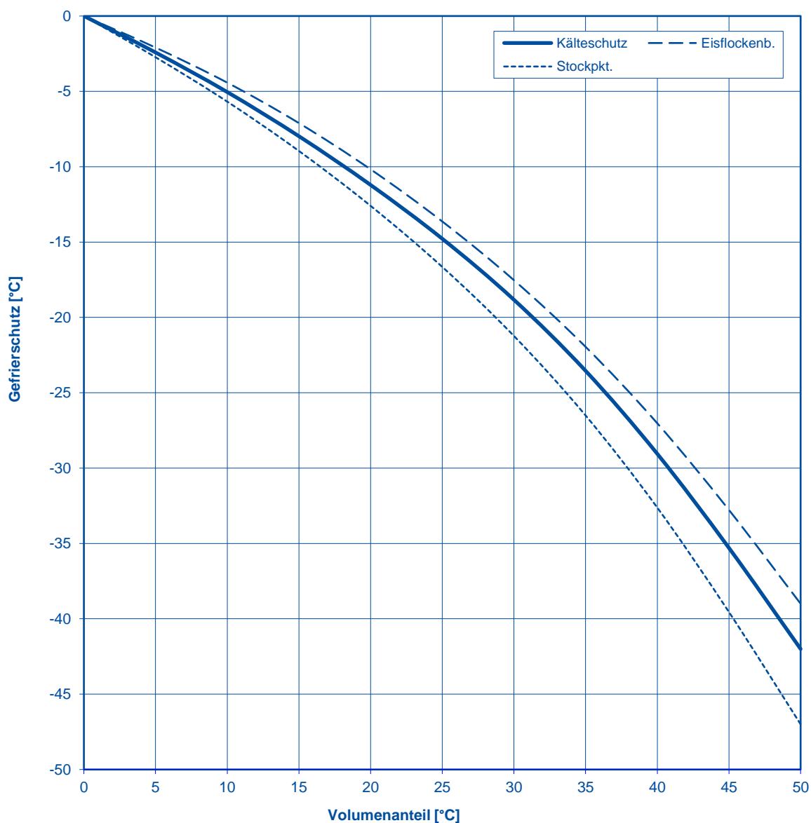
Abhängigkeit des Kälteschutz wässriger MAINTAIN FRICOFIN Mischungen
